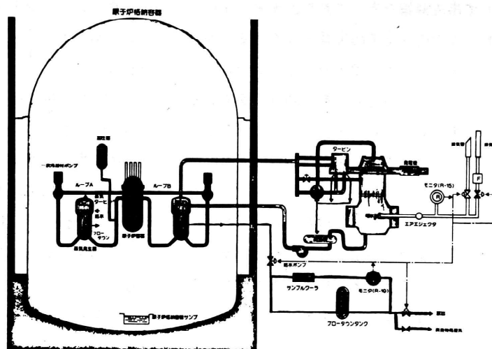
第1図 主系統説明図
